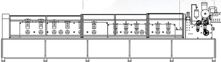
滾輪成型主機 Roll Forming Section
