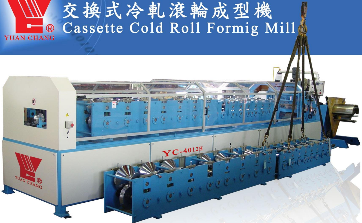
滾輪成型主機 Roll Forming Section
