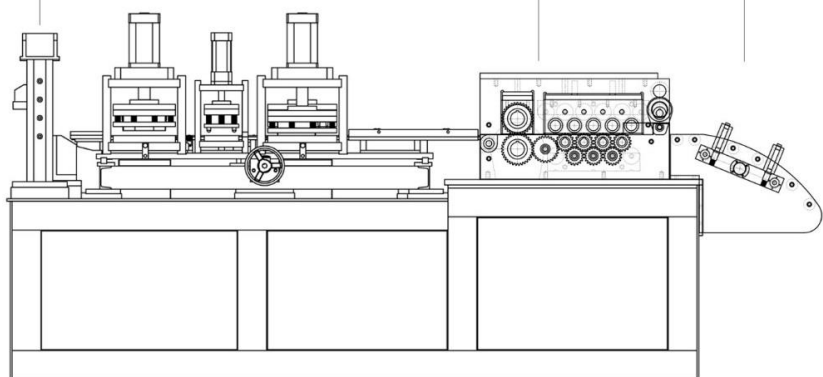
切斷機 Cutting Machine
